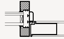
DEKO DG - DOUBLE GLAZED DOOR
