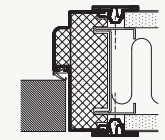
DEKO TD - SOLID TIMBER DOOR
