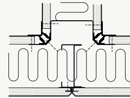
T-CONNECTION
