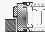
DEKO TD - SOLID TIMBER DOOR
